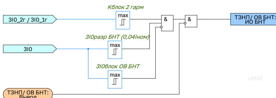
Рисунок 2.39 – Функциональная схема логики органа выявления БНТ
