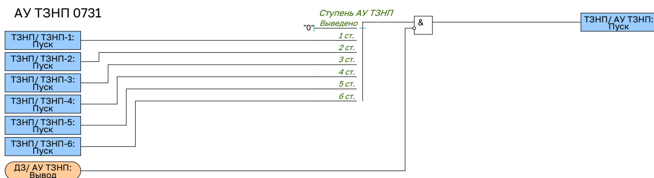
Рисунок 2.43 – Функциональная схема пуска АУ ТЗНП
