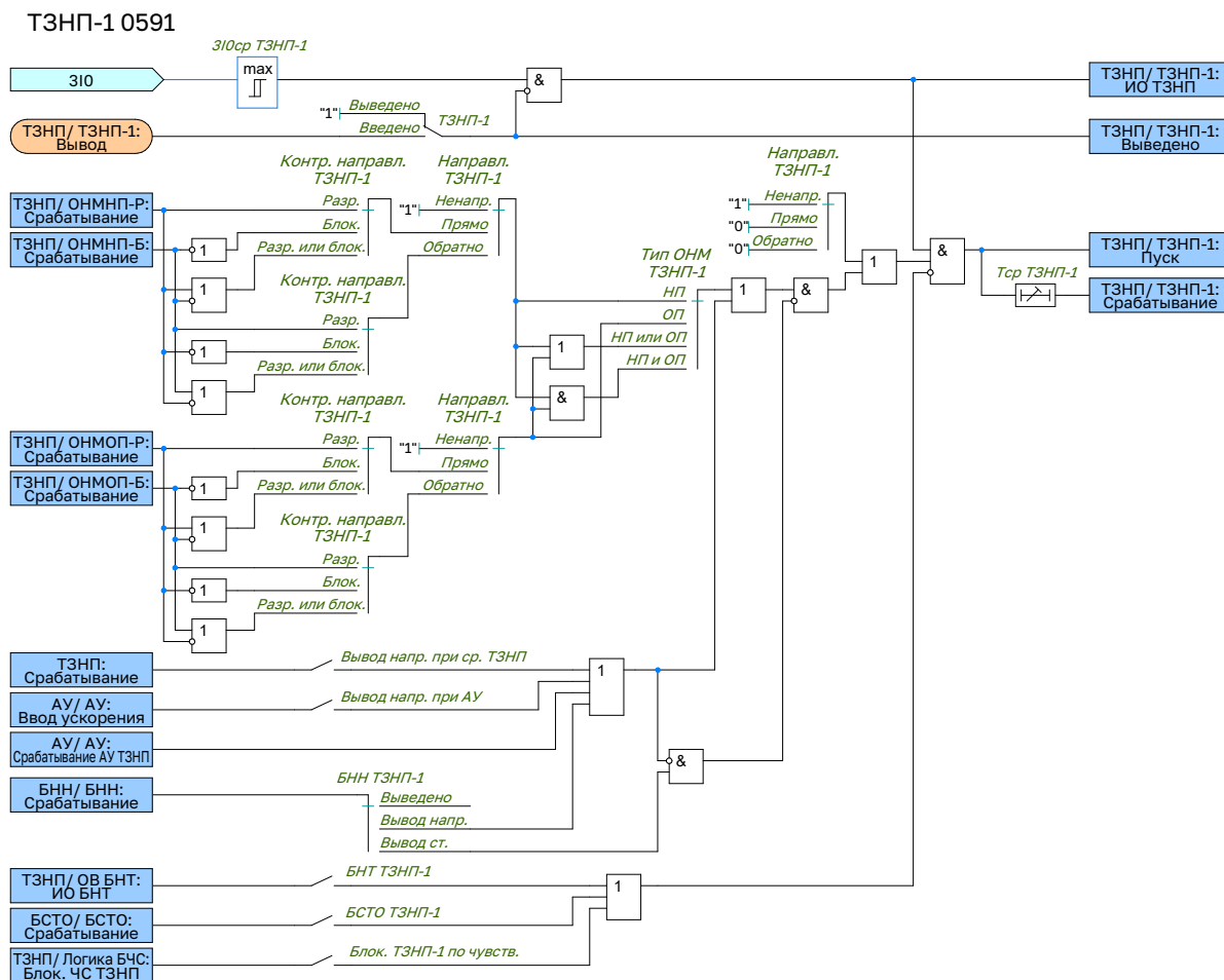
Рисунок 2.38 – Функциональная схема ступени ТЗНП-1
