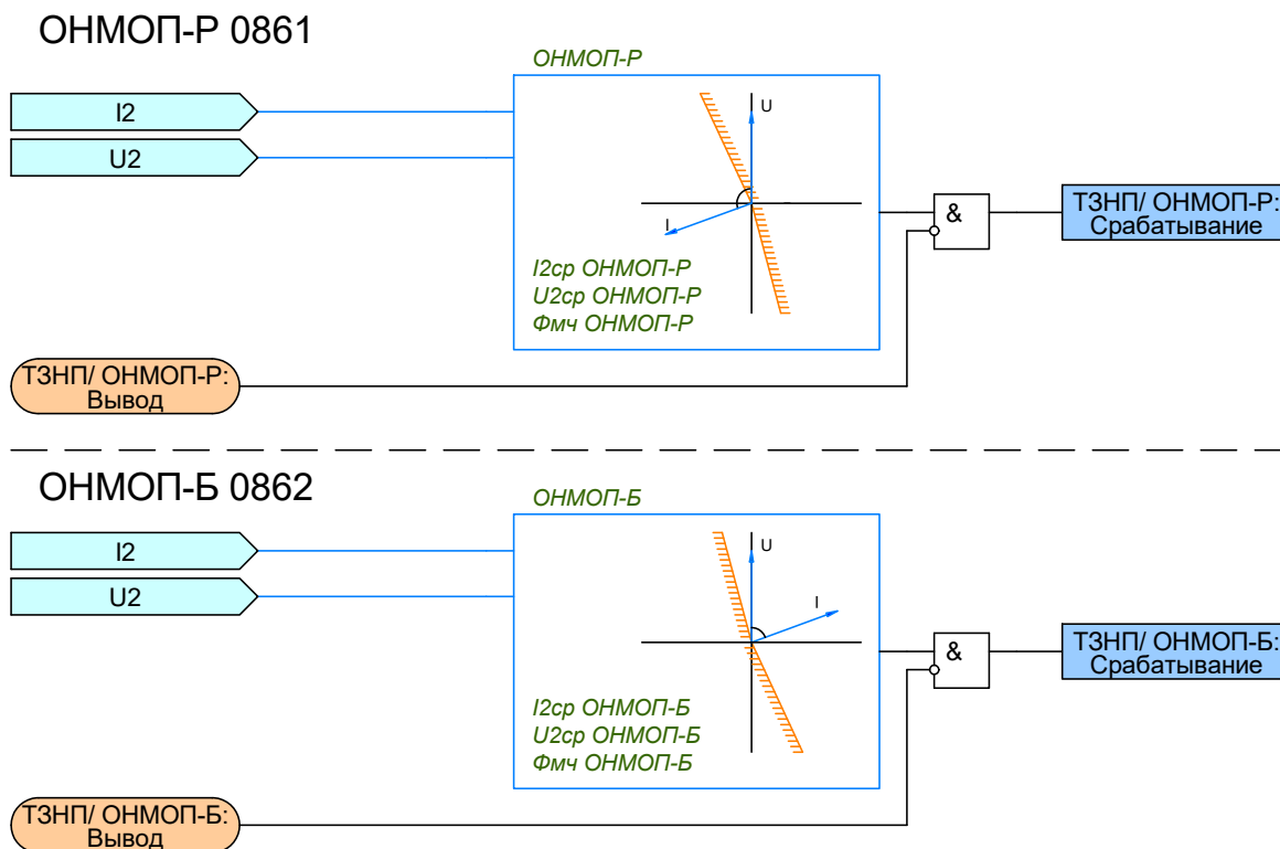
Рисунок 2.42 – Функциональная схема логики ОНМОП
