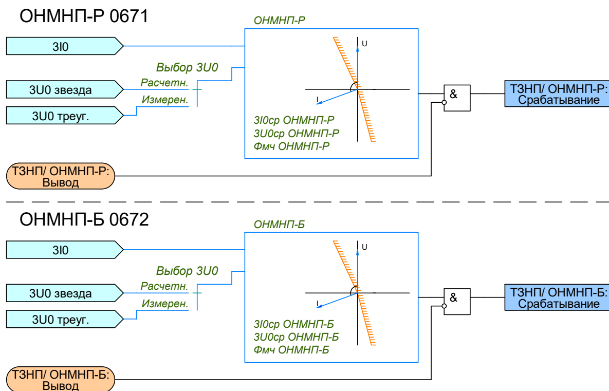
Рисунок 2.41 – Функциональная схема логики ОНМНП
